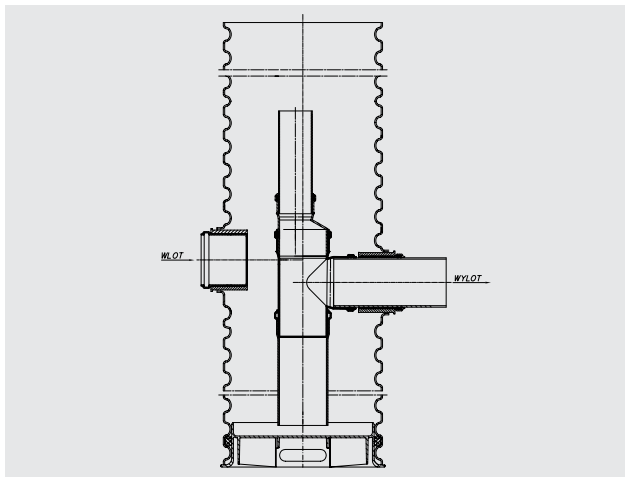
Rys. 35. Budowa studzienki Azura (z filtrem DN 110)
