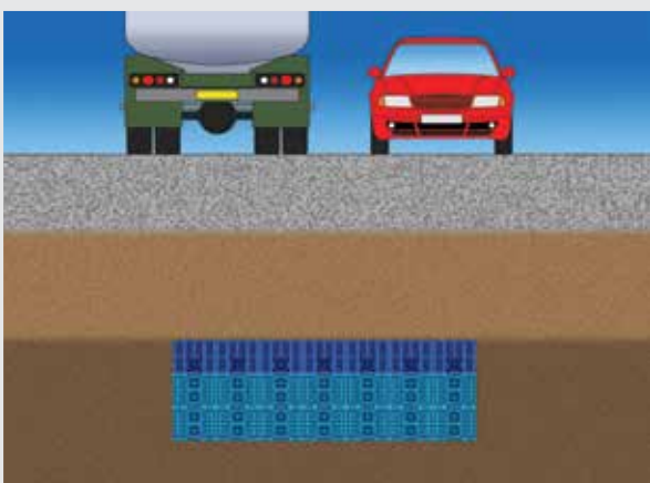
Rys. 15. Przykładowe obszary zastosowań skrzynek Wavin AquaCell Plus
