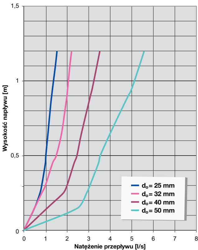
Rys. 22. Wykres wydajności regulatora Wavin Orifice
