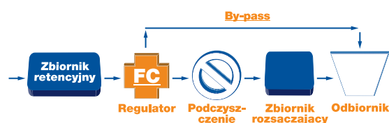
Rys. 20. Obejście by-passowe systemu podczyszczania
