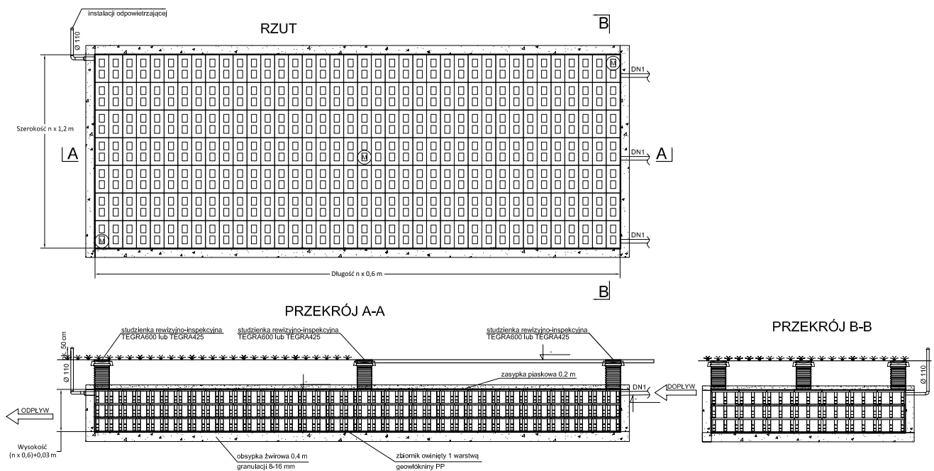
Rys. 26. Przykład zbiornika retencyjno-rozsączającego Wavin Q-Bic Plus, ułożonego w trzech warstwach
