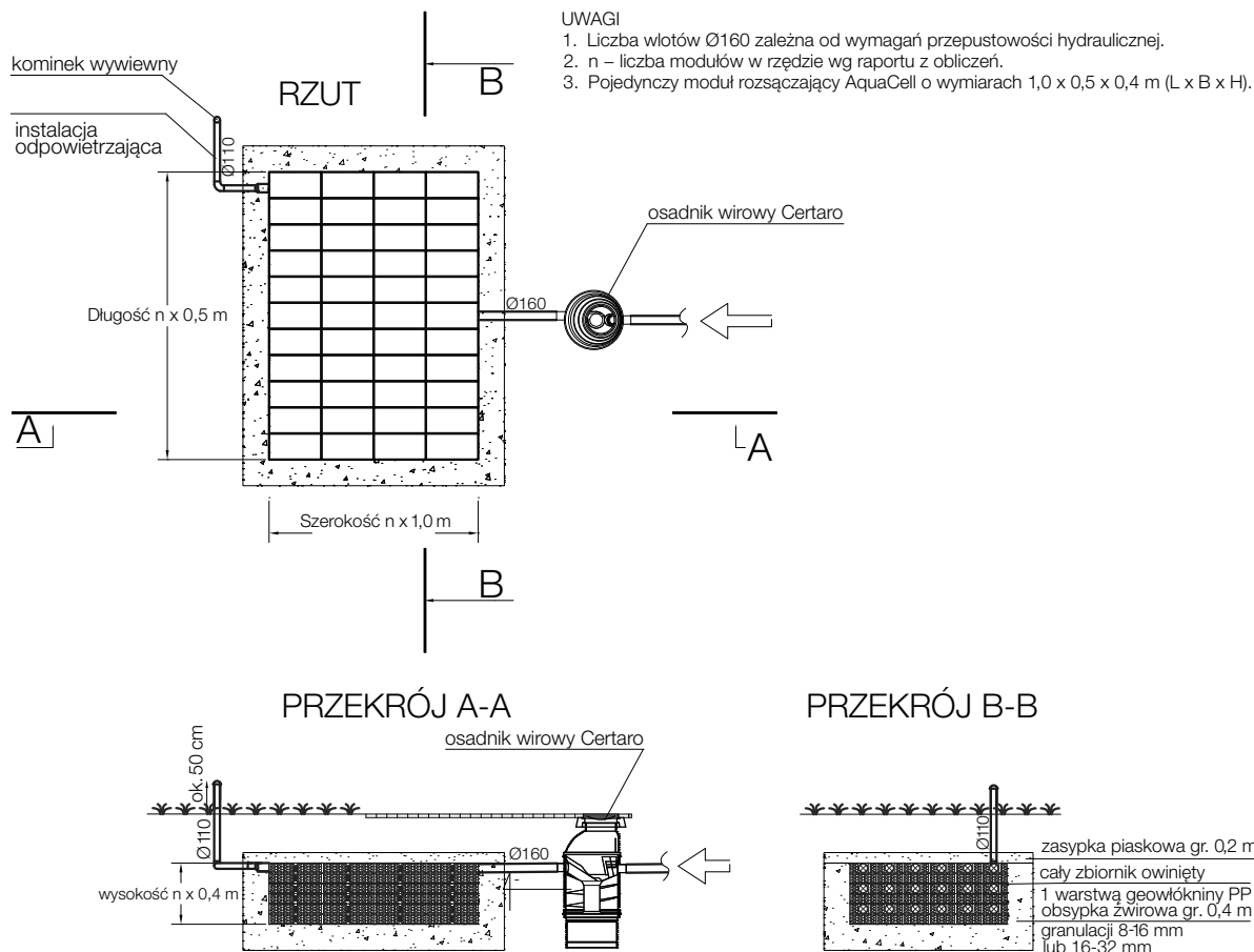
Rys. 25. Ogólny schemat zabudowy zbiornika retencyjno-rozsączającego Wavin AquaCell w zabudowie wielowarstwowej z osadnikiem wirowym Wavin Certaro
