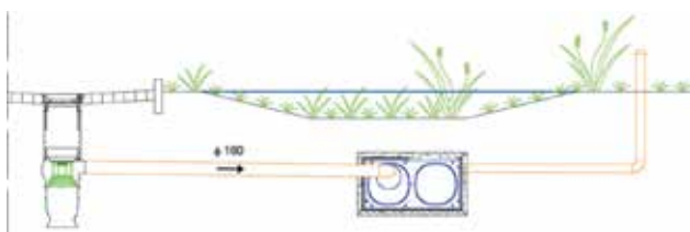
Rys 3. Zbiornik retencyjno-rozsączający z możliwością inspekcji i czyszczenia współpracujący z Tegra RG, umieszczony pod niecką z nasadzoną roślinnością
