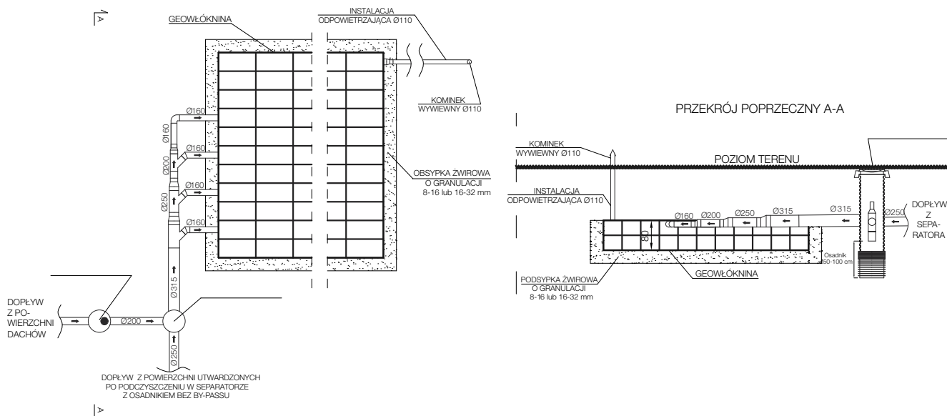
Rys. 24. Ułożenie skrzynek Wavin AquaCell w dwóch warstwach. Odpowietrzezenie poprzez rurę wywiewną
