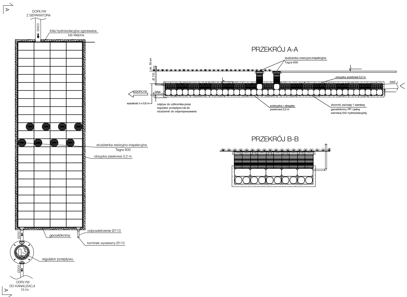
Rys. 27. Przykład zbiornika retencyjnego opartego na Wavin Q-Bic/Wavin Q-BB
