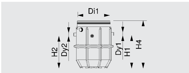
Rys. 41. Wymiary separatora Certaro NS 3
