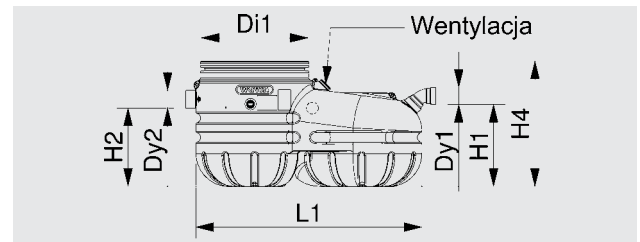
Rys. 42. Wymiary separatora Certaro NS 6 i Certaro NS 10
