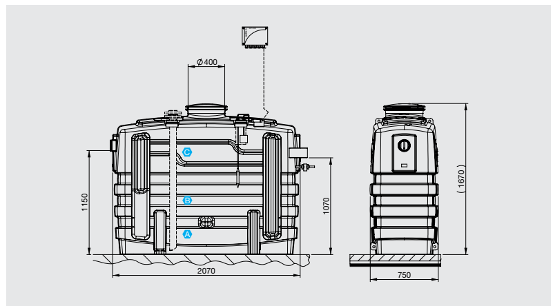
Rys. 51. Wymiary separatora EuroREK NS4 SL
