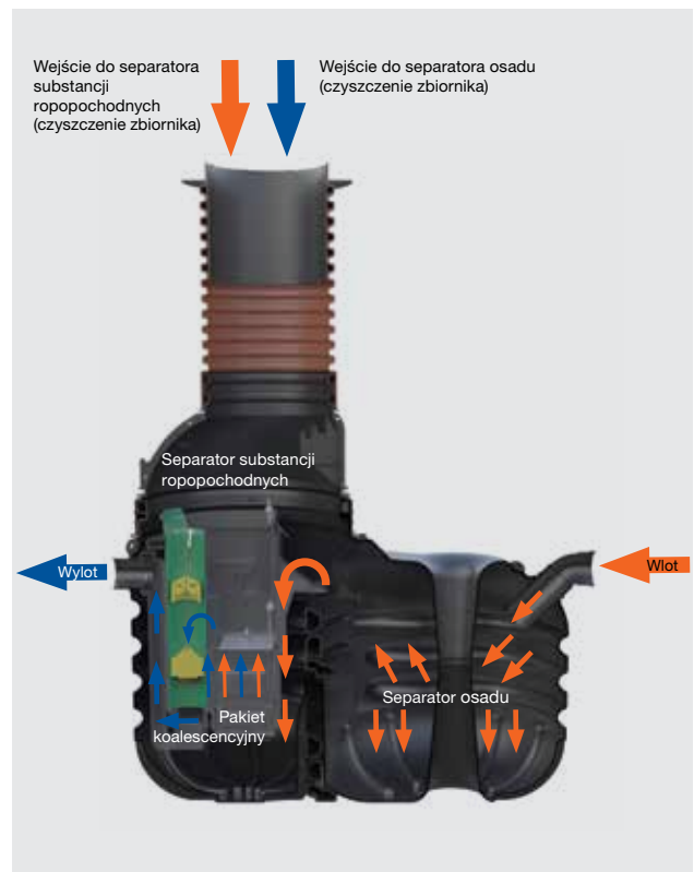
Rys. 40. Zasada działania separatora Wavin NS
