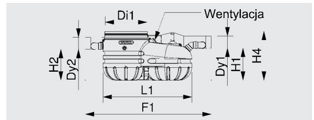
Rys. 44. Wymiary separatora Certaro NS 6 by-pass i Certaro NS 10 by-pass
