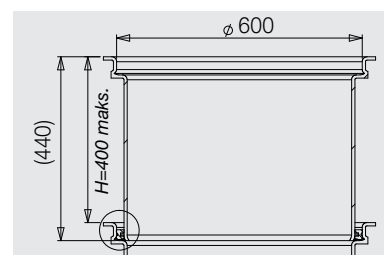
Rys. 54. Nadstawka do separatora MiniPEK 0,3
