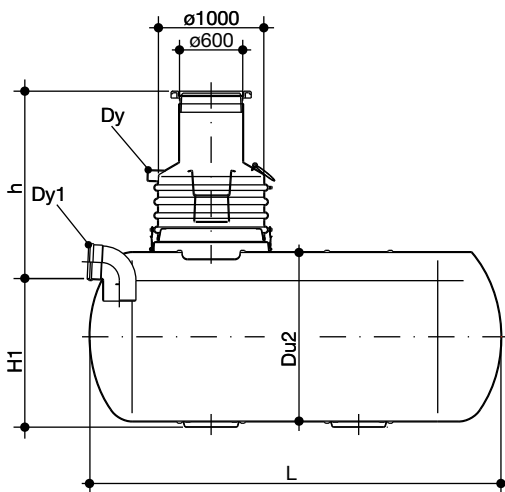
Rys. 31. Podstawowe wymiary zbiornika z GRP
