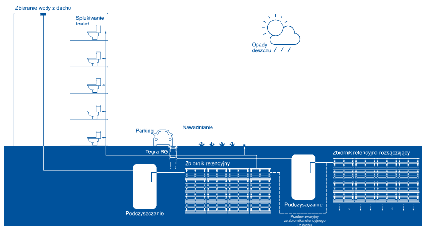
Rys 9. Zbieranie wody z powierzchni utwardzonych z wykorzystaniem ponownym wody deszczowej. Dodatkowo przelew awaryjny do zbiornika retencyjno-rozsączającego
