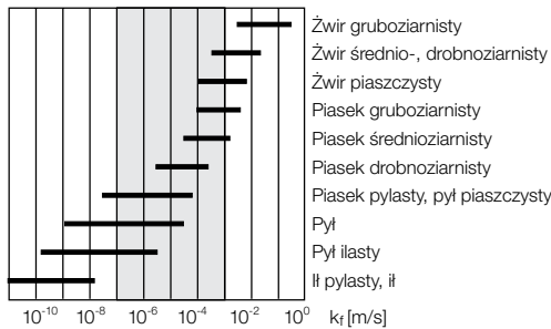
Rys. 2. Współczynnik przepuszczalności skał klastycznych i zakres infiltracji
