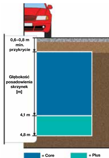
Rys. 13. Maksymalne głębokości posadowienia skrzynek Wavin AquaCell w zależności od rodzaju obciążenia powierzchni
