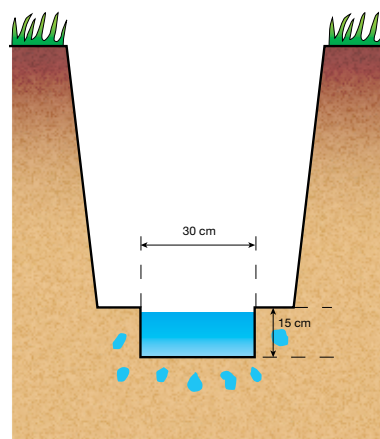
Rys. 1. Model testu perkolacyjnego
