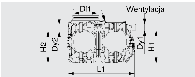
Rys. 43. Wymiary separatora Certaro NS 15 i Certaro NS 20
