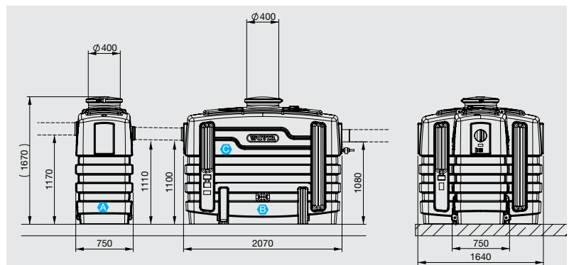
Rys. 52. Wymiary separatora EuroREK NS7 SL
