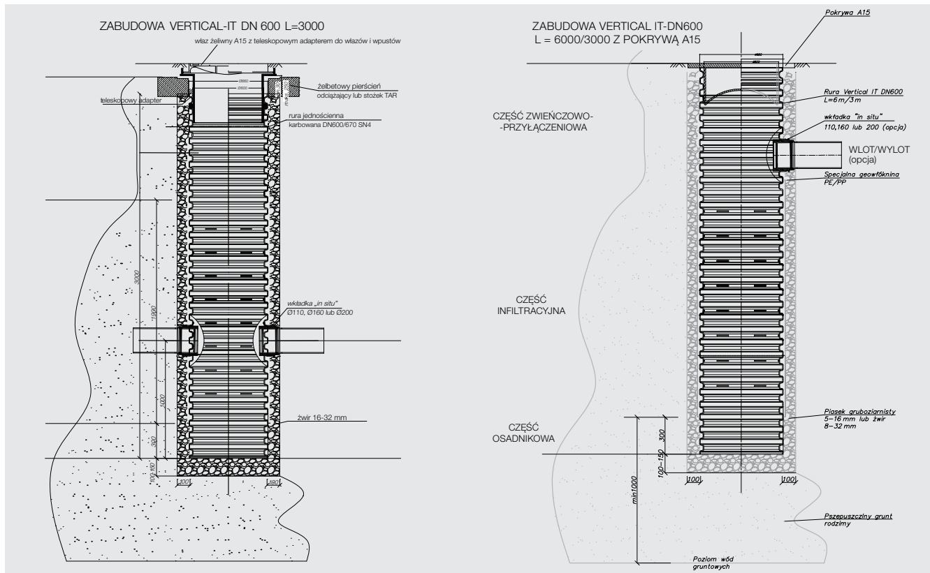
Rys. 29. Przykładowe ułożenie rur Vertical IT pod pasem zieleni
