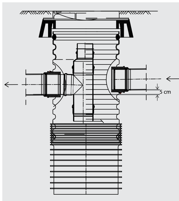
Rys. 36. Studzienka osadnikowa Tegra 600 z filtrem Azura 200
