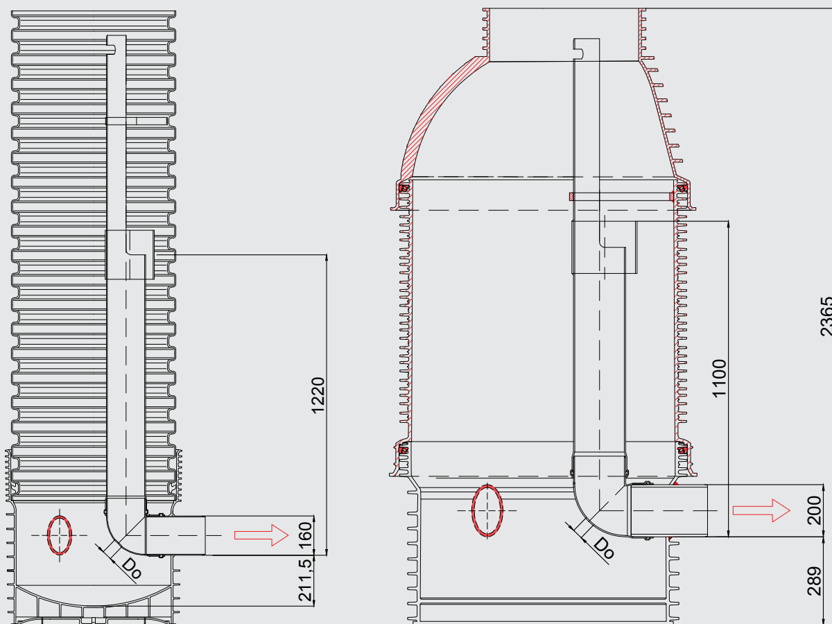
Rys. 21. Regulator Orifice w obudowie studni Tegra 600 i Tegra 1000 IG
