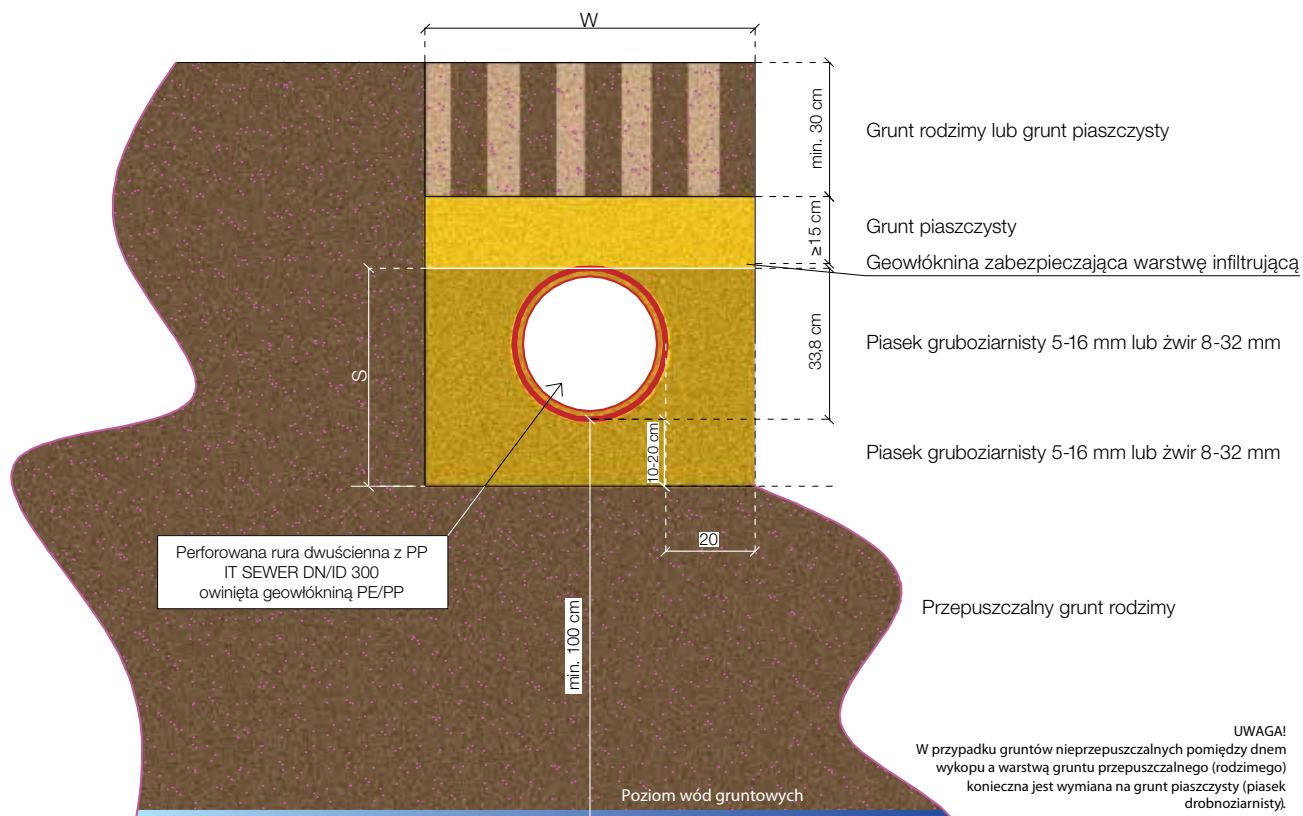
Rys. 28. Przykładowe ułożenie rur IT Sewer pod pasem zieleni
