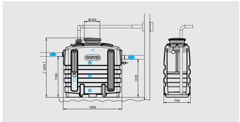
Rys. 50. Wymiary separatora EuroREK NS2 SL
