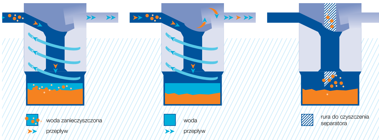
Rys. 38. Zasada działania Certaro HDS Pro
