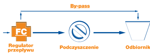
Rys. 19. Ograniczenie przepływu przez filtr lub separator
