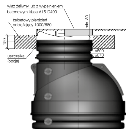
Właz A15, B125 lub D400 na żelbetowym pierścieniu
