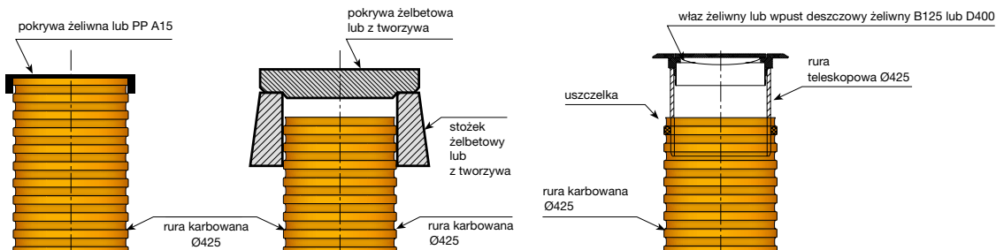
Pokrywa A15 na rurze karbowanej
