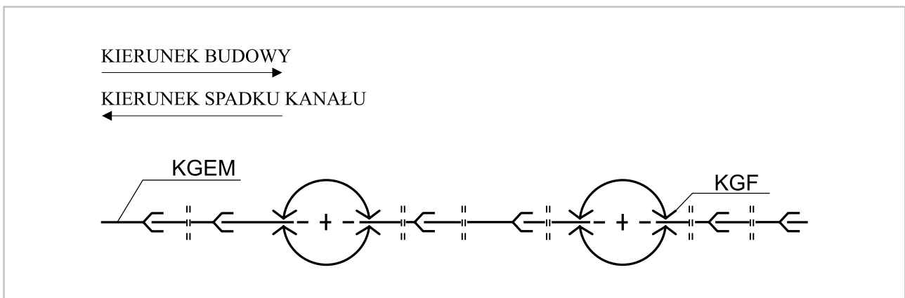
Rys. 21. Łączenie rur KG ze studzienkami z tworzyw sztucznych wykonanych fabrycznie z kielichami na dopływie i odpływie
