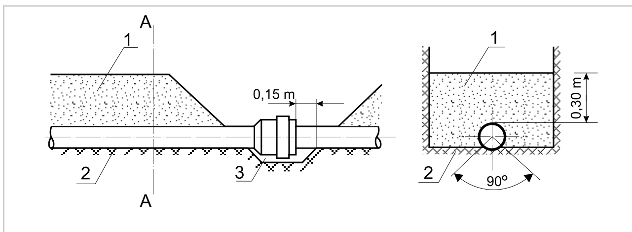
Rys.18. Układanie rur kanalizacyjnych w gruntach zwięzłych
